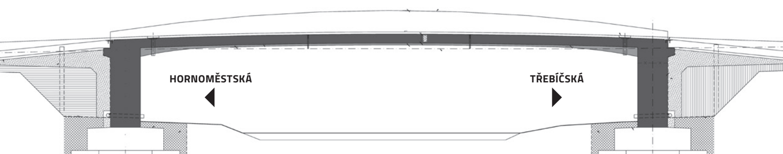
Podélný řez novým mostem
