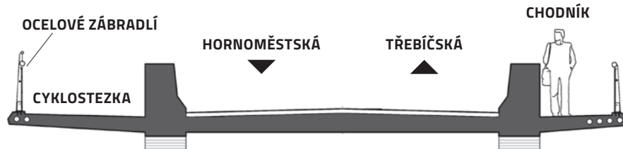
Příčný řez novým mostem
